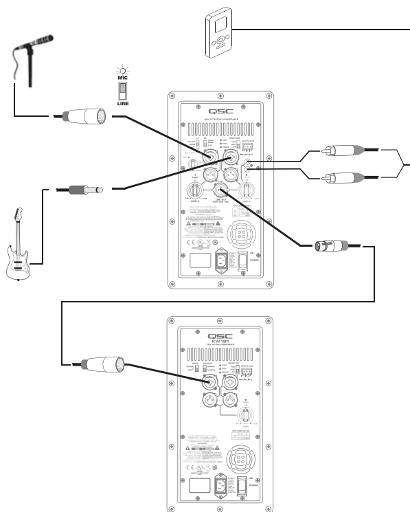
Типовая схема передачи смешанного сигнала от независимой аудиосистемы после усиления в KW 181
