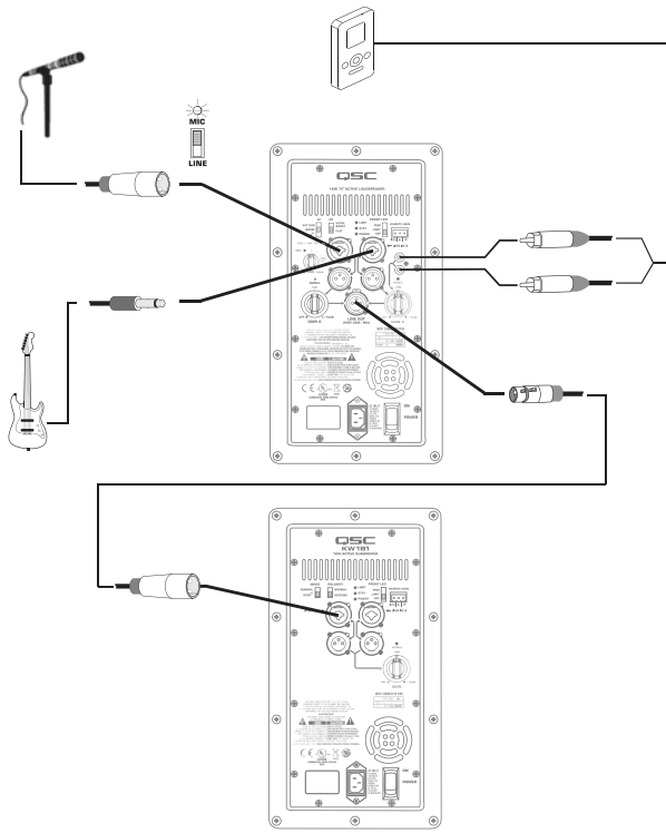
نظام صغير قائم بذاته شائع يمرر الإشارة التي تصدر من المزج بين مقويات الإشارة (Gain A + B) إلى KW 181
