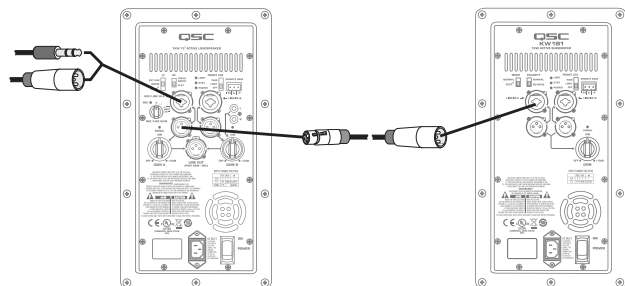
Передача сигнала в KW 181
