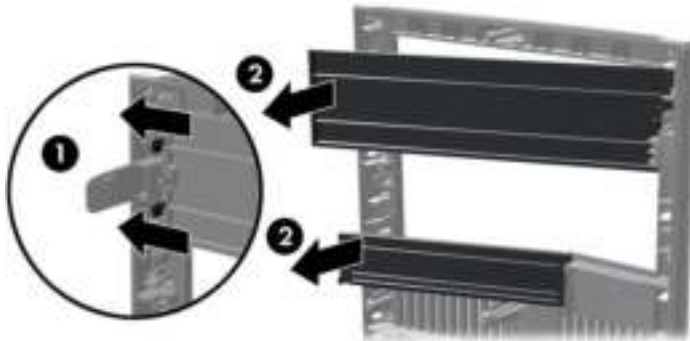
Afbeelding 3-5 Afdekplaatje verwijderen
