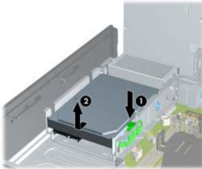
Afbeelding 4-36 Vaste schijf verwijderen
