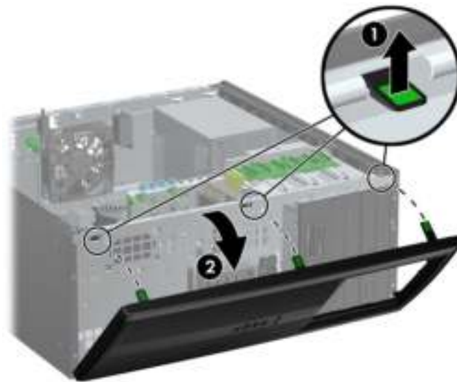
Afbeelding 2-3 Voorpaneel verwijderen
