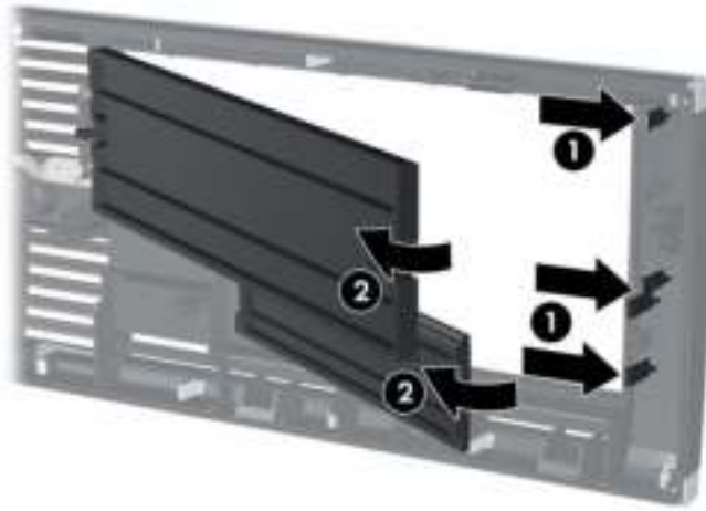
Afbeelding 4-4 Afdekplaatje verwijderen
