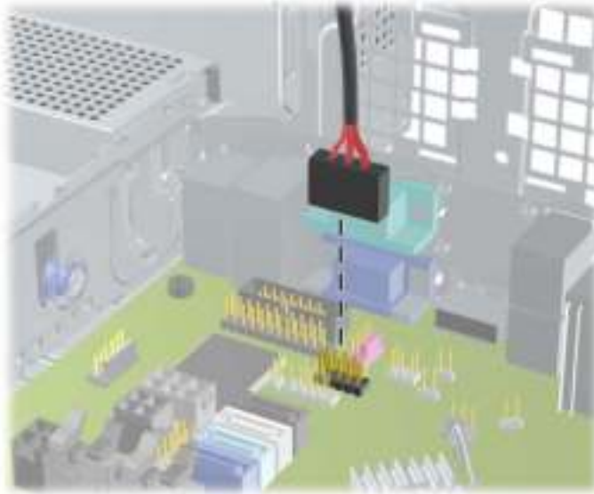
Afbeelding 4-27 USB-kabel van de mediakaartlezer ontkoppelen
