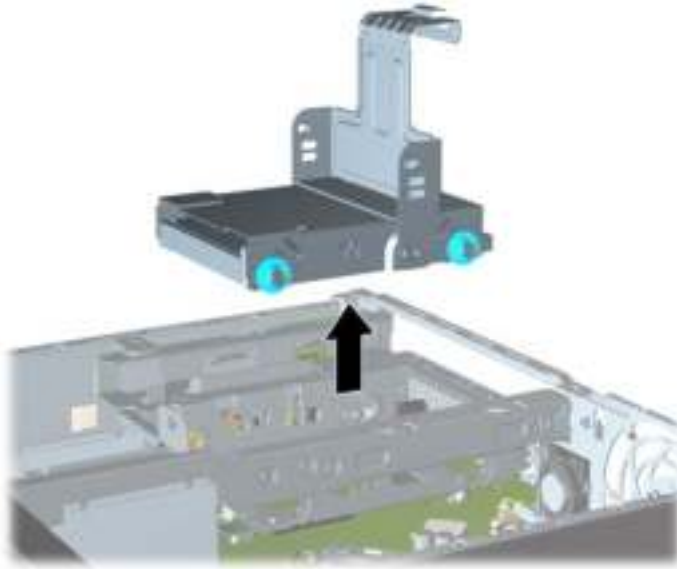
Afbeelding 5-16 Houder van de vaste schijf verwijderen
