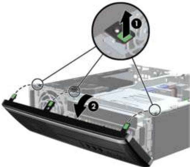
Afbeelding 5-4 Voorpaneel verwijderen
