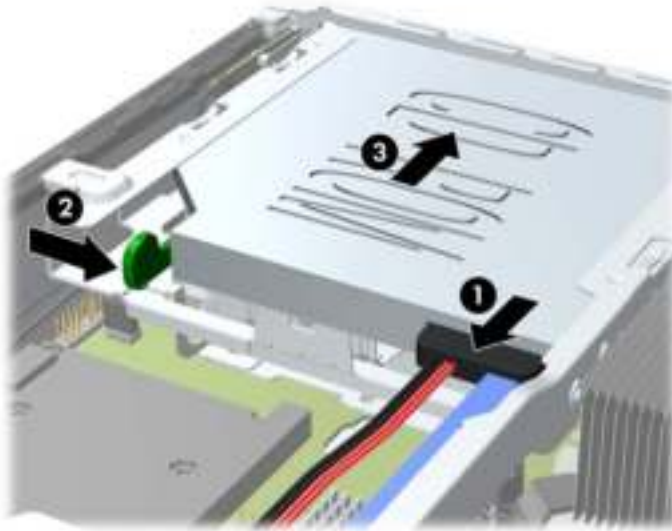
Afbeelding 5-12 Optischeschijfeenheid verwijderen
