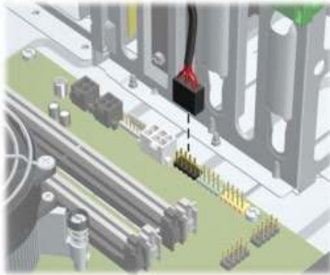
Afbeelding 2-15 USB-kabel van de mediakaartlezer ontkoppelen
