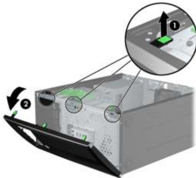
Afbeelding 3-4 Voorpaneel verwijderen
