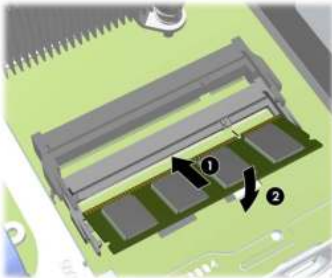
Afbeelding 5-11 SODIMM installeren
