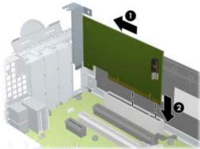
Afbeelding 4-14 Uitbreidingskaart installeren
