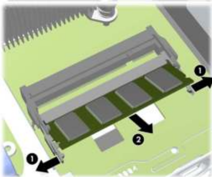
Afbeelding 5-10 SODIMM verwijderen
