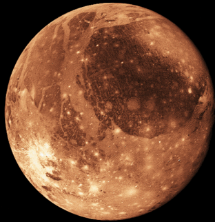
Ganymede 5262 km
