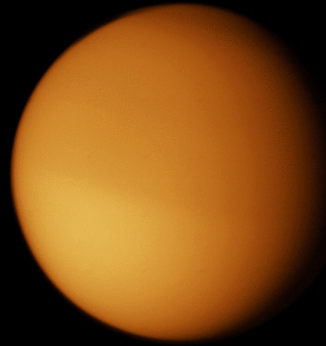
Titan 5150 km
