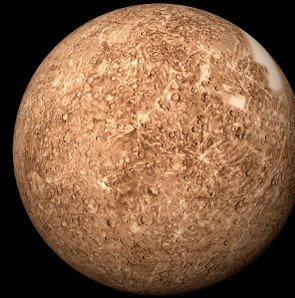
Mercury 4880 km
