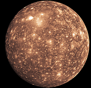
Callisto 4806 km
