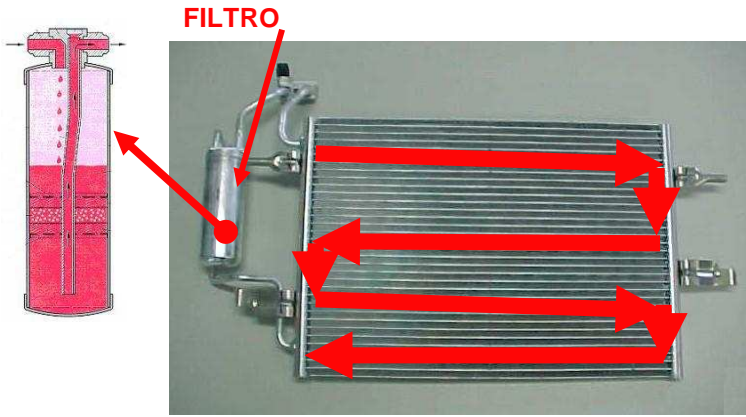
Condensador brasado convencional. Filtro secador remoto.
