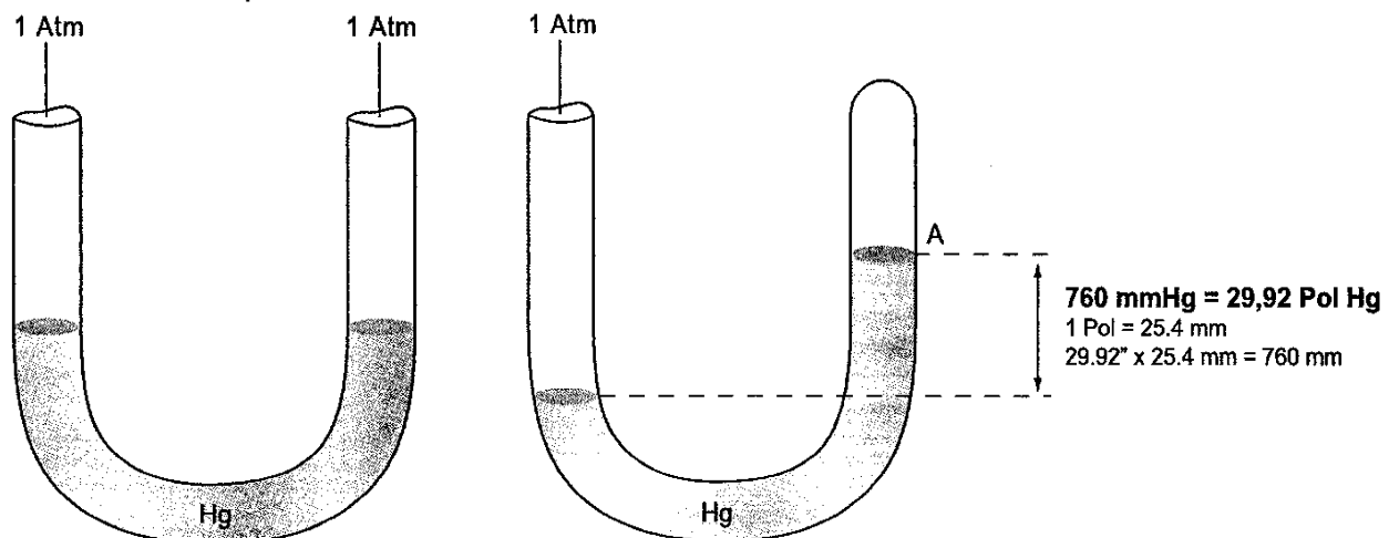
Fig.45 Barômetro equalizado
